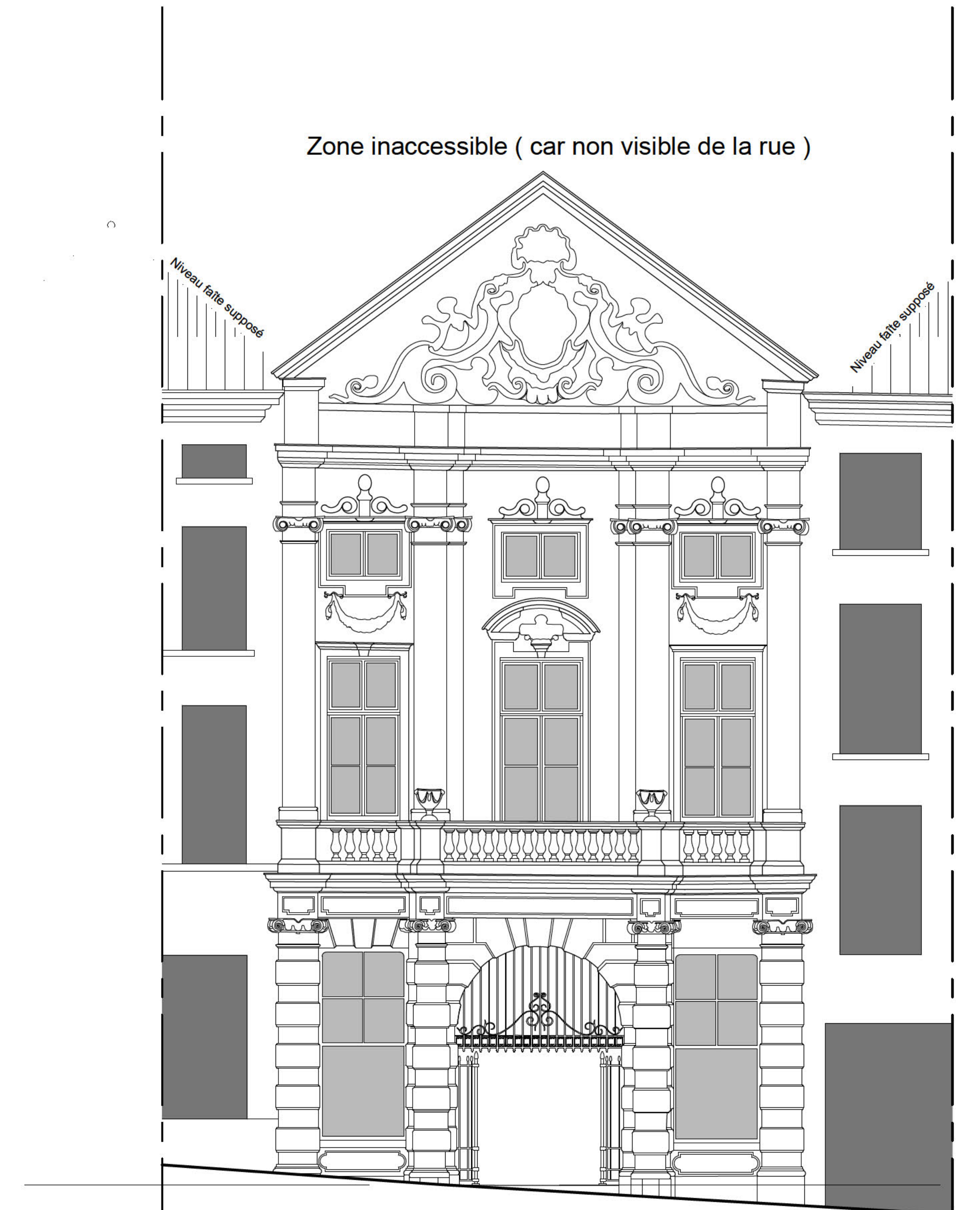
Façade B-B ( Rue de la madeleine )
